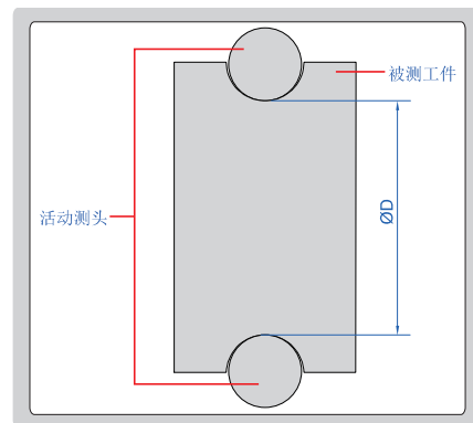
测量球轴承沟道直径 \varnothing D
